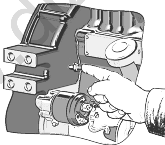
Рисунок 20 - Установка фиксатора в отверстие заднего листа и маховика.
