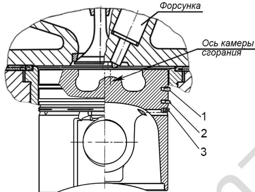
Рисунок 27 - Схема установки поршневых колец
