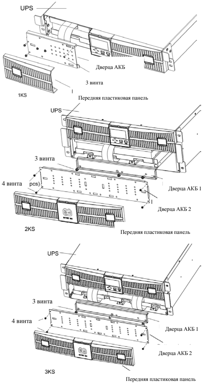
Рис.7-1 Снятие передней пластиковой крышки лицевой панели и крышки батарейного блока
