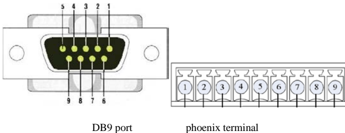
Рис 5- 1: Сухой контакт
