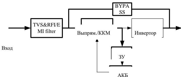
Рис. 1- 5: Режим байпаса
