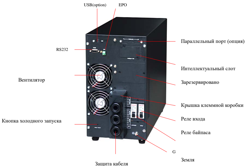
Рис. 1- 2: Вид сзади
