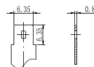
Вывод Ш-6,35
