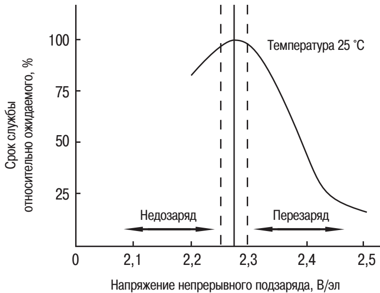
Рис. 14 Зависимость срока службы аккумулятора от напряжения подзаряда.
